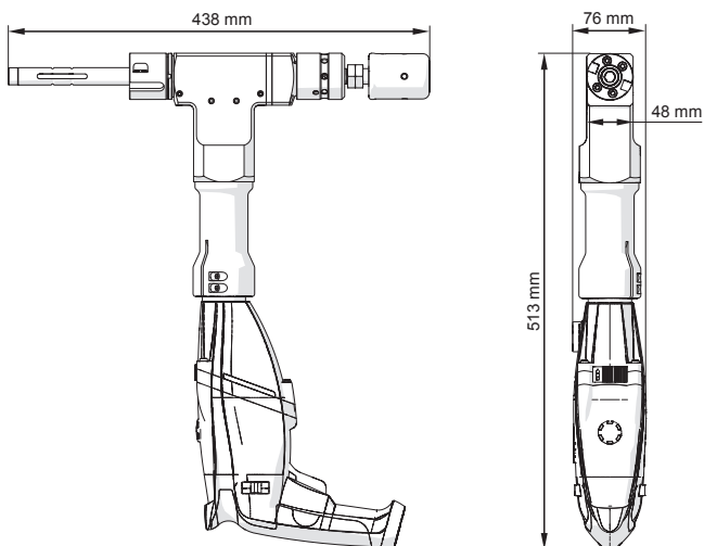
PRO 2 PB con motor eléctrico
