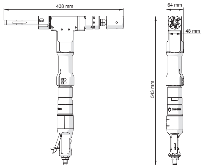
PRO 2 PB con motor neumático
