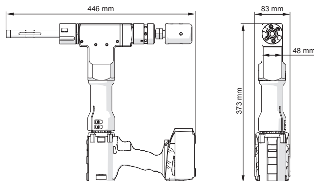
PRO 2 PB con motor a batería
