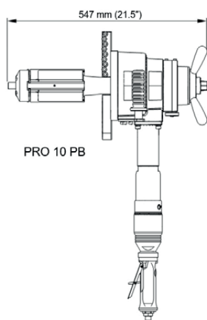
PRO 10 PB con motor neumático
