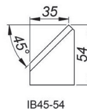
Cuchilla de Corte Bisel interior 45° Altura 54mm. [IB45/54] Referencia: NOZ-000026
