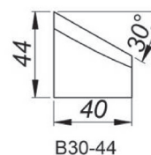
Cuchilla de Corte Bisel 30° Altura 44mm. [B30/44] Referencia: NOZ-000018
