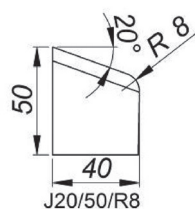
Cuchilla de Corte bisel Tipo J 20° Altura 50mm. Radio 8mm. [J20/50/R8] Referencia: NOZ-000016
