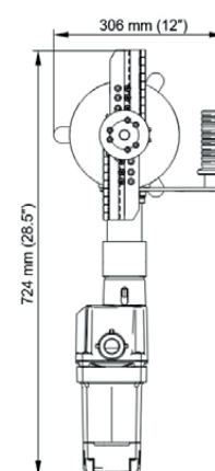
PRO 10 PB con motor eléctrico
